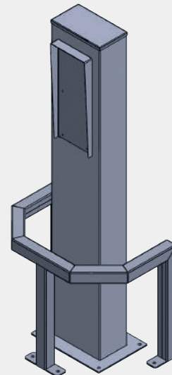
Arçeau de Protection pour borne APB001
