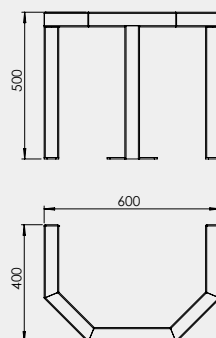
Arçeau de Protection pour borne APB001
